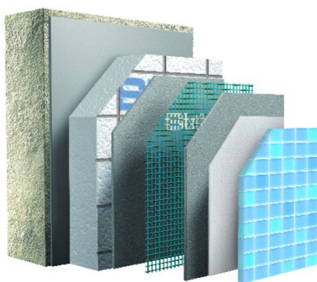
Systeemopbouw 300T-Ceramique
